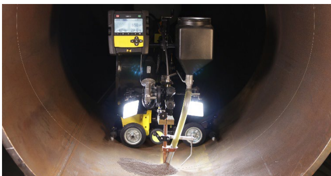
Traktor Versotrac w wersji z 3 kołami z opcjonalnym zestawem lamp LED
